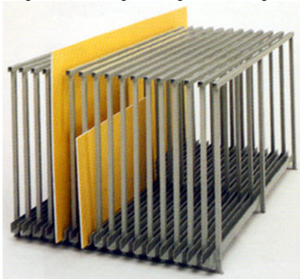
Skivställ MODELL A, här med 16 fack. Höjd 950 mm. Bredd: 1225 mm. Djup: 1900 mm. Fler eller färre fack = +/- 75 mm i bredd
